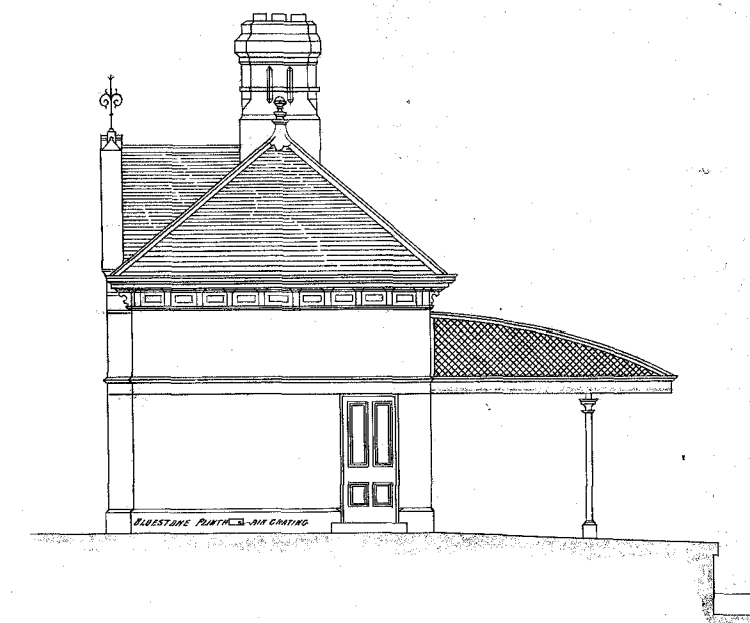
END ELEVATION
